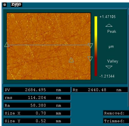
ケメット鉄定盤+9μダイヤモンドスラリー
