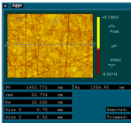
ケメット銅定盤+3μダイヤモンドスラリー
