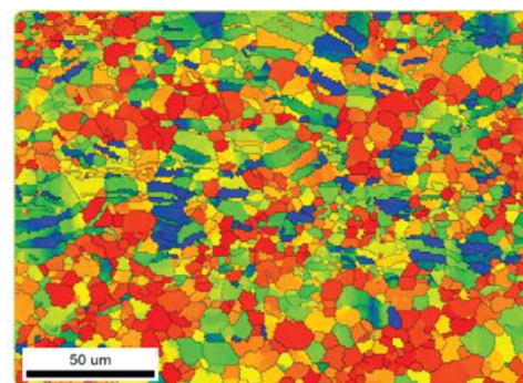
EBSD mapping
